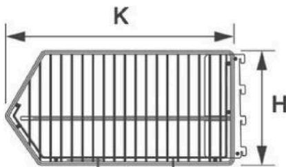
Корзина навесная | Basket Hinged
